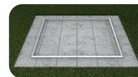
Aluminium-Bodenrahmen auflegen.
