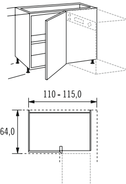
Eckunterschrank, 1 Drehtür
