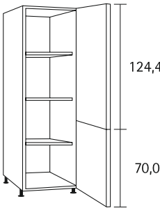
Hochschrank, 2 Drehtüren
