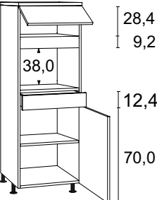
Midischränk für Mikrowelle, 1 Klappe, 1 Schubkasten, 1 Drehtür 37 41 AL B 60,0 cm H 170,0 - 177,6 cm T 55,5 cm
