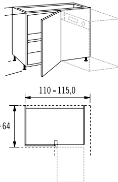
Eckunterschrank, 1 Drehtür
