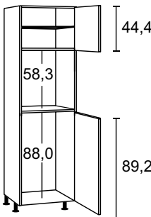
Hochschrank für Backofen und Kühlschrank, 2 Drehtüren 45 47 AS B 60,0 cm H 205,2 - 212,8 cm T 55,5 cm
