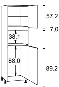
Hochschrank für Mikrowelle und Kühlschrank, 2 Drehtüren 45 47 AT B 60,0 cm H 205,2 - 212,8 cm T 55,5 cm
