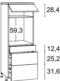
Midischränk für Backofen, 1 Klappe, 1 Schubkasten, 2 Auszüge 37 42 23 AM B 60,0 cm H 170,0 - 177,6 cm T 55,5 cm
