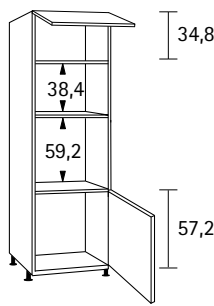
Hochschrank für Mikrowelle und Backofen, 1 Klappe, 1 Drehtür 45 52 AR B 60,0 cm H 205,2 - 212,8 cm T 55,5 cm
