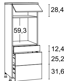
Midischrank für Backofen, 1 Klappe, 1 Schubkasten, 2 Auszüge
