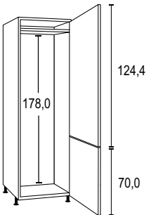
Hochschrank für Kühl-/Gefrierschränk, 2 Drehtüren 45 49 A0 B 60,0 cm H 205,2 - 212,8 cm T 55,5 cm
