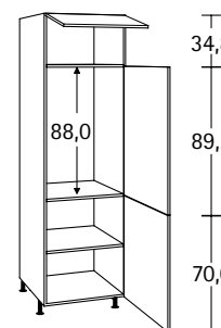
Hochschrank für Kühlschrank, 1 Klappe, 2 Drehtüren
