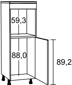
Midischränk für Kühlschrank und Backofen, 1 feste Blende, 1 Drehtür 37 40 AK B 60,0 cm H 170,0 - 177,6 cm T 55,5 cm
