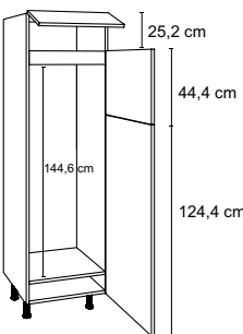
Hochschrank für Kühl-/Gefrierkombination, 1 Klappe, 2 Drehtüren 45 53 AU B 60,0 cm H 205,2 - 212,8 cm T 55,5 cm
