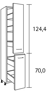
Apothekerschränk, 2 Auszüge mit oben 3 und unten 2 Schubkästen 50 51 AQ B 30,0 cm H 205,2 - 212,8 cm T 55,5 cm
