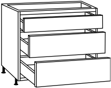
Unterschränk mit 1 Schubkasten, 2 Auszügen
