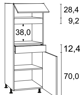
Midischrank für Mikrowelle, 1 Klappe, 1 Schubkasten, 1 Drehtür
