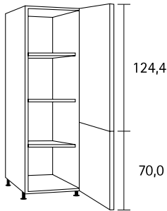
Hochschrank, 2 Drehtüren 45 46 A0 B 60,0 cm H 205,2 - 212,8 cm T 55,5 cm
