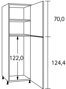
Hochschrank für Kühlschrank, 2 Drehtüren 45 48 A0 B 60,0 cm H 205,2 - 212,8 cm T 55,5 cm
