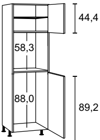
Hochschrank für Backofen und Kühlschrank, 2 Drehtüren
