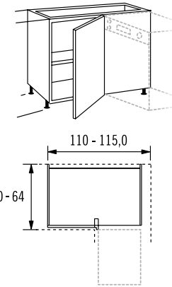
Eckunterschränk, 1 Drehtür
