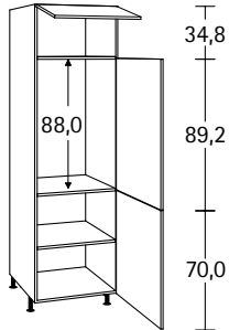
Hochschrank für Kühlschrank, 1 Klappe, 2 Drehtüren 45 47 AP B 60,0 cm H 205,2 - 212,8 cm T 55,5 cm
