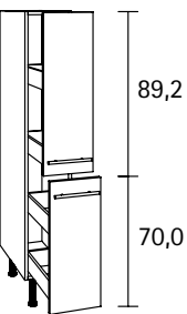
Midi-Apothekerschränk, 2 Auszüge mit je 2 Schubkästen 43 44 AN B 30,0 cm H 170,0 - 177,6 cm T 55,5 cm
