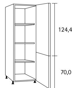
Hochschrank 2 Drehtüren
