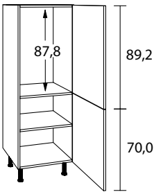
Midischränk für Kühlschrank, 2 Drehtüren 37 39 AJ B 60,0 cm H 170,0 - 177,6 cm T 55,5 cm
