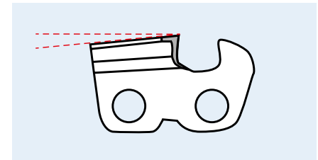
Zahndach fällt nach hinten ab
