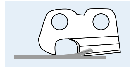
Hobelzahnprinzip
