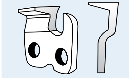
Vollmeißelzahn
