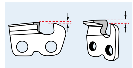
Tiefenbegrenzerabstand
