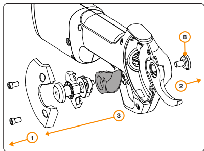
Kuva 8. Leikkuuterän vaihtaminen. Seuraa numerorjärjestystä.
