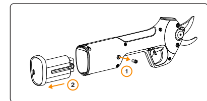
Rysunek 6. Wyjmowanie i wymiana akumulatora.
