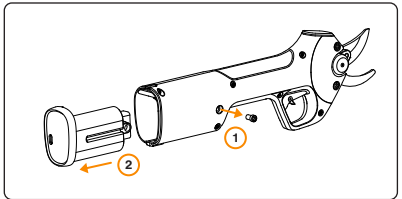
6. ábra. Az akkumulátor eltávolítása és cseréje.
