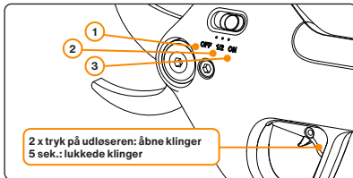
Illustration 4: Tænd/sluk-knappens forskellige trin og åbning af klingen.
