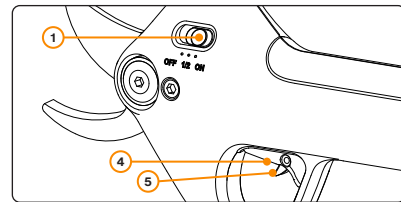
3. ábra: A főkapcsoló (1), a kioldókapcsoló (4) és a biztonsági kioldó (5).
