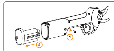
Joonis 6. Aku eemaldamine ja vahetamine.
