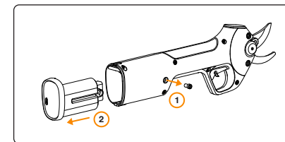
Obrázok 6. Vybratie a výmena akumulátora.
