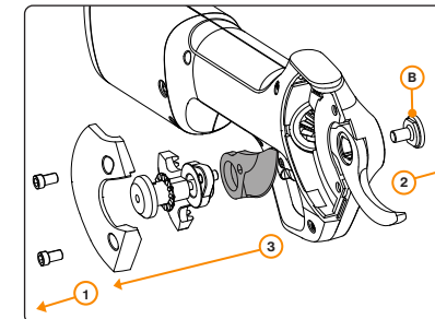
Joonis 8. Lõiketera vahetamine. Järgige numbritest järjestust.
