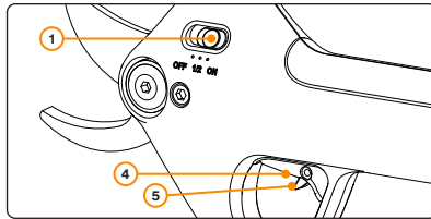
3 pav. Maitinimo jungiklis (1), paleidiklio jungiklis (4) ir apsauginis paleidiklis (5).
