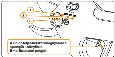
4. ábra: A főkapcsoló és a pengeszétnyitás különböző szakaszai.
