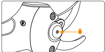
5. ábra. A kenőnyílás helye.
