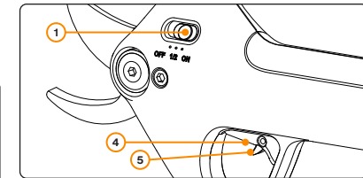
Figur 3: Strømbryter (1), utløserbryter (4) og sikkerhetsutløser (5).
