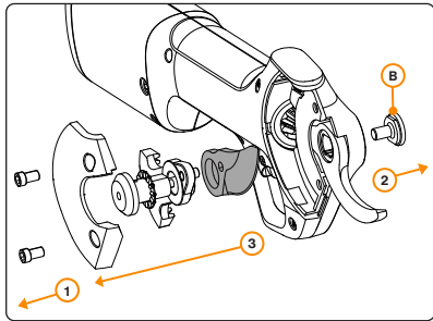
Obrázok 8. Výmena rezacej čepele. Postupujte podľa číselného poradí.
