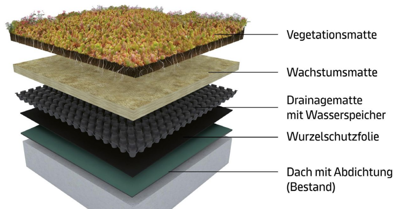
Lieferumfang des Urbanscape Gründach-Set:
