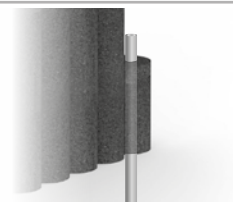
Montagerohr, Art.-Nr. 251110991 Ø 33,7 mm, Länge: 500 mm
