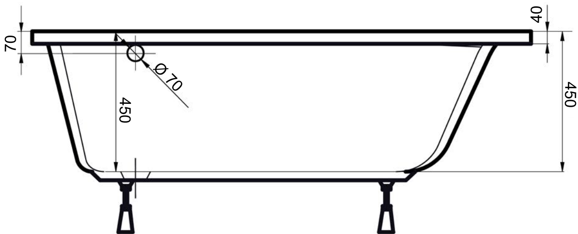
Modell B - Linke Hand entspricht spiegelverkehrter Ausführung
