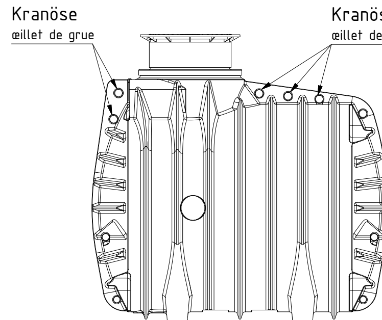
Ansicht von links vue de gauche
