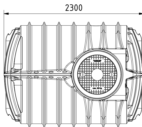
Ansicht von oben vue du dessus
