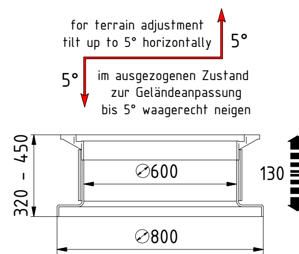
Ansicht von links vue de gauche
