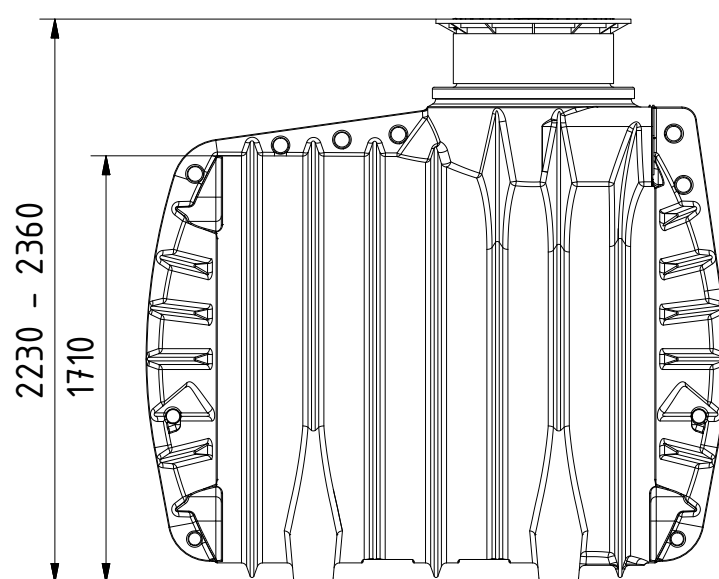
Ansicht von rechts vue de droit
