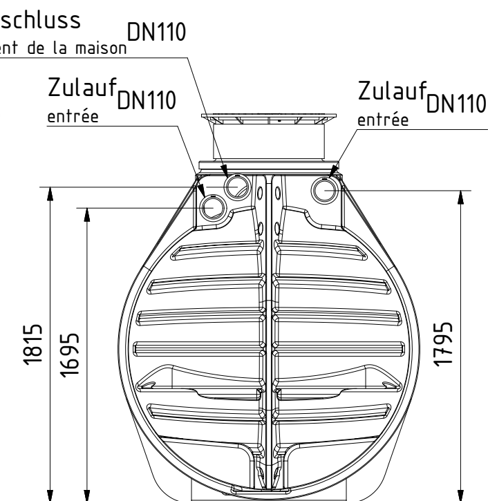
Ansicht von hinten vue de derrière
