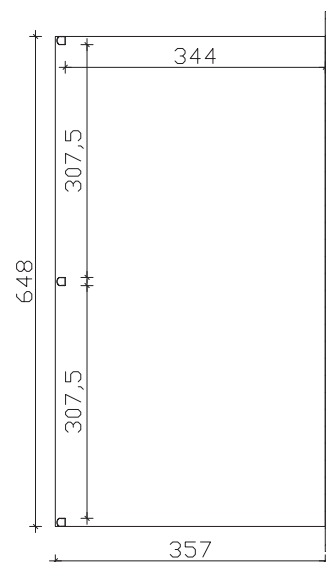
Grundriss
