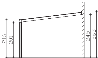
Schnitt
