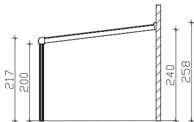
Schnitt
