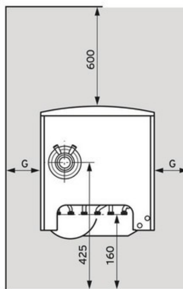
Draufsicht
