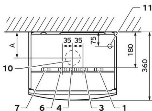
Draufsicht (Anschlüsse im Gerät)
