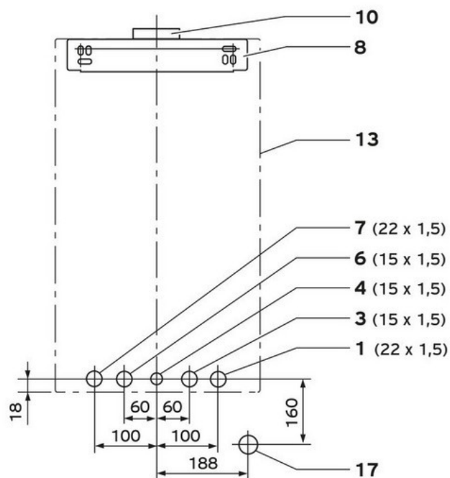
Neu-Installation Unterputz (Stichmaße Aufputz identisch)
