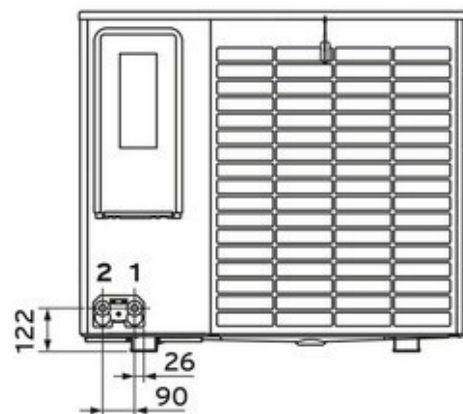
Rückansicht aroTHERM plus
