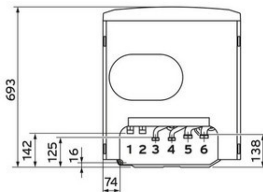
Draufsicht uniTOWER
