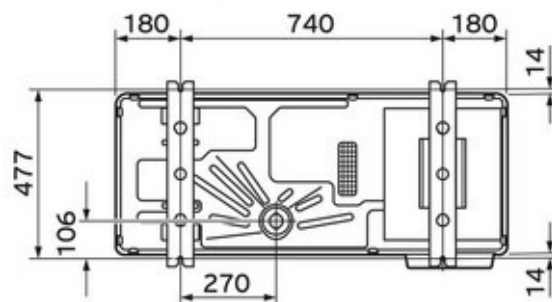
Unteransicht aroTHERM plus
