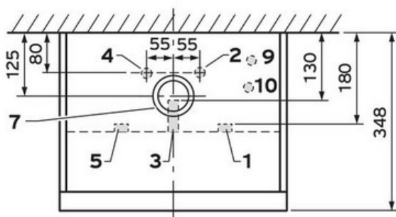
Draufsicht (Anschlüsse im Gerät)
