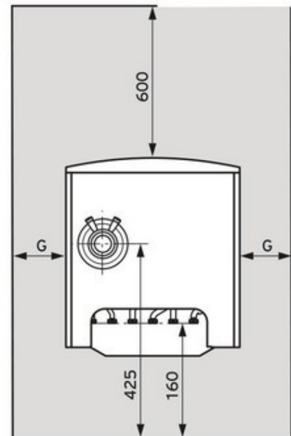
Draufsicht
