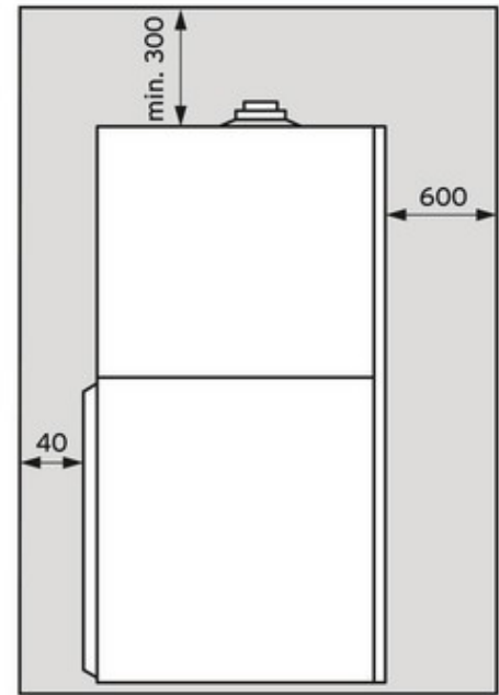
Seitenansicht
