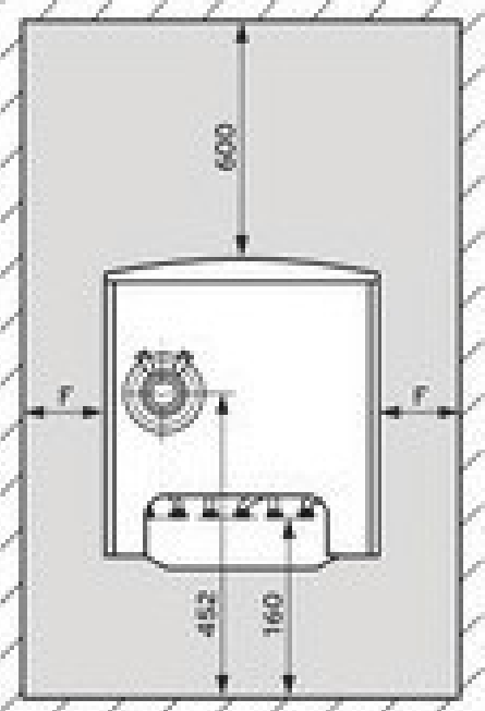
Draufsicht
