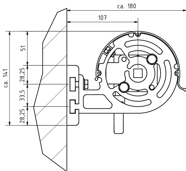
Seitenansicht Fassadenmarkise Typ A und Typ S
