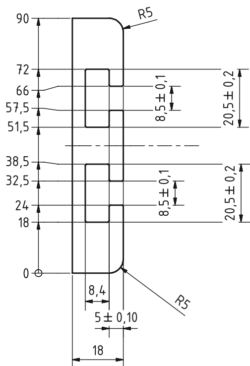
Konsole für Wandmontage Typ A und Typ S
