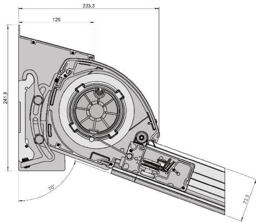
Seitenansicht Wandmontage in mm
