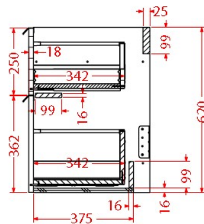
SEZIONE A-A
