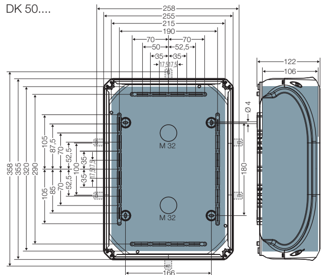
DK 50....
