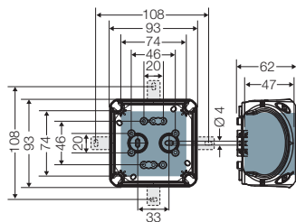
KF 02.. G/B
