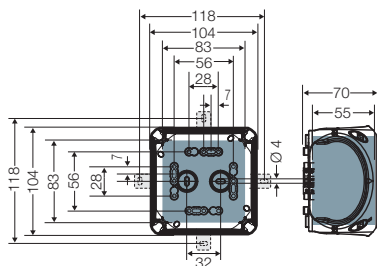
KF 04.. G/B
