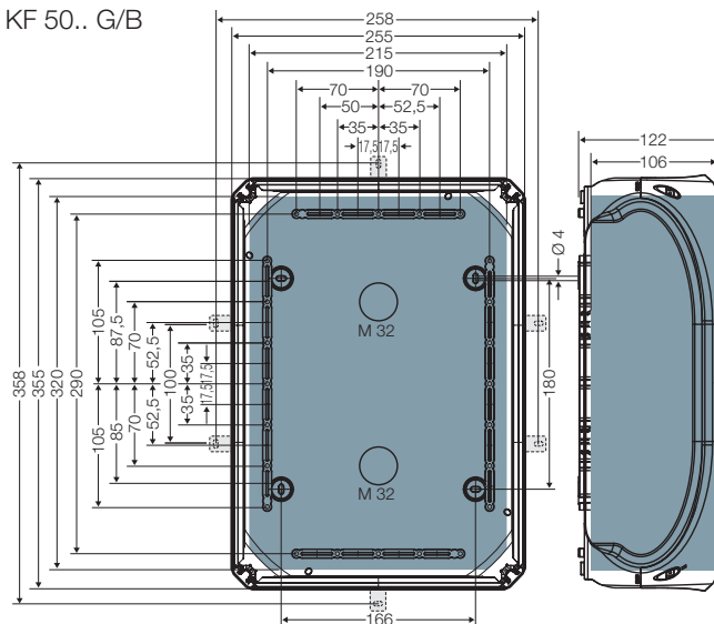
KF 50.. G/B
