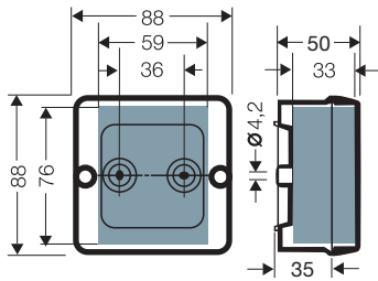
DE 932.
