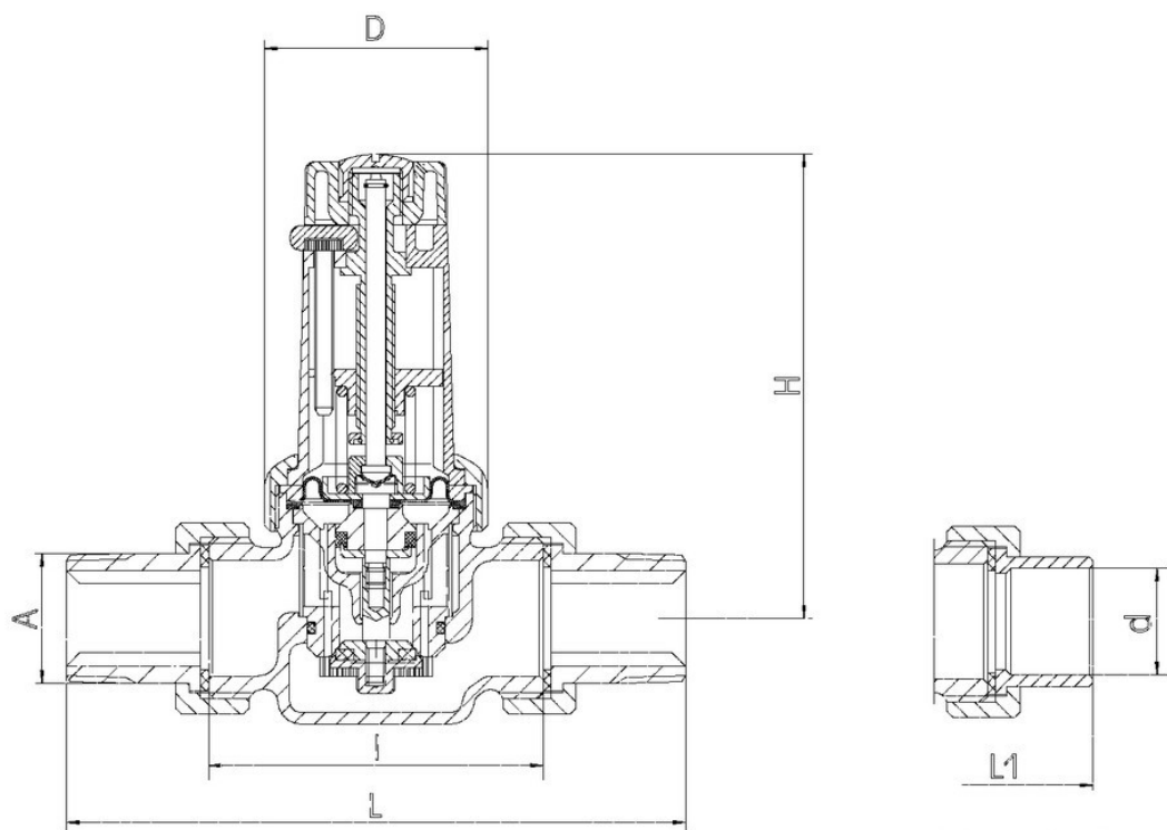
Lötverschraubung
