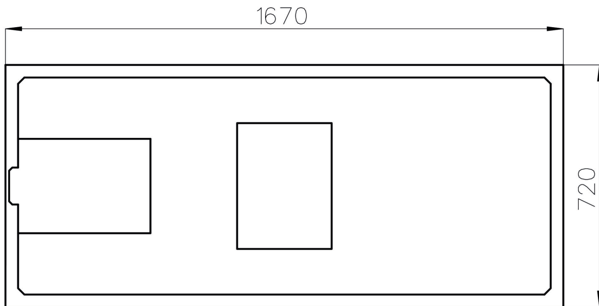
Draufsicht
