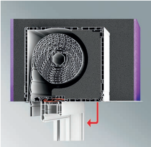
Typ A-Elite XT – Revision* innen unten Abbildung inkl. Putzträgerplatte beidseitig Kasten innen eckig Putzträger innen und außen möglich
