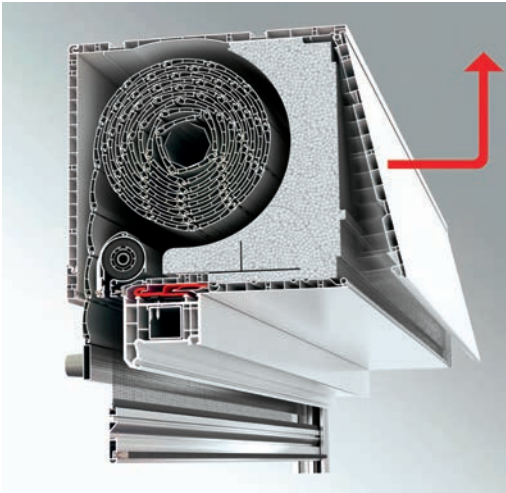
Typ A-Elite XT – Revision* innen hinten Kasten innen eckig Putzträger außen möglich
