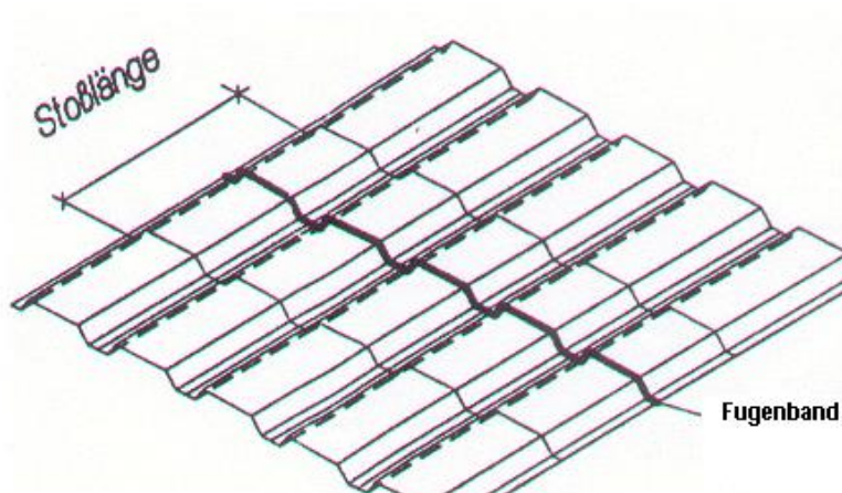
Detail: Plattenstoß
