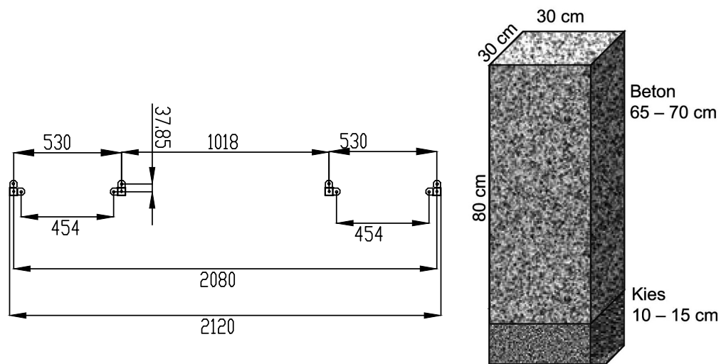
FUNDAMENT
