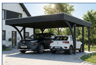
350346-16-40 Carport Friesland Set H, 546 x 555 cm, mit zwei Einfahrtsbögen, anthrazit
