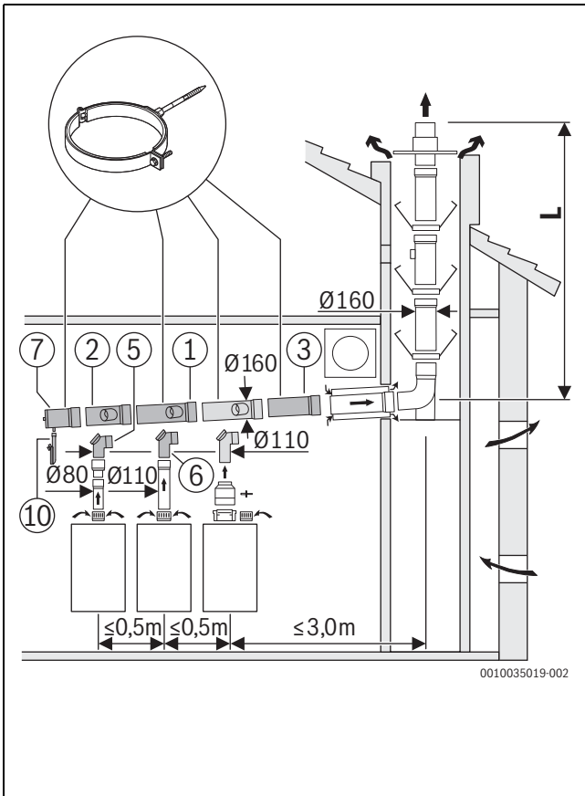
12 DN160 - DN160
