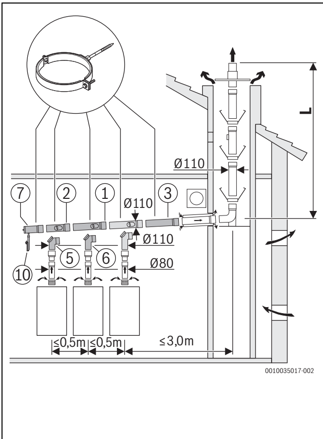
10 DN110 - DN110
