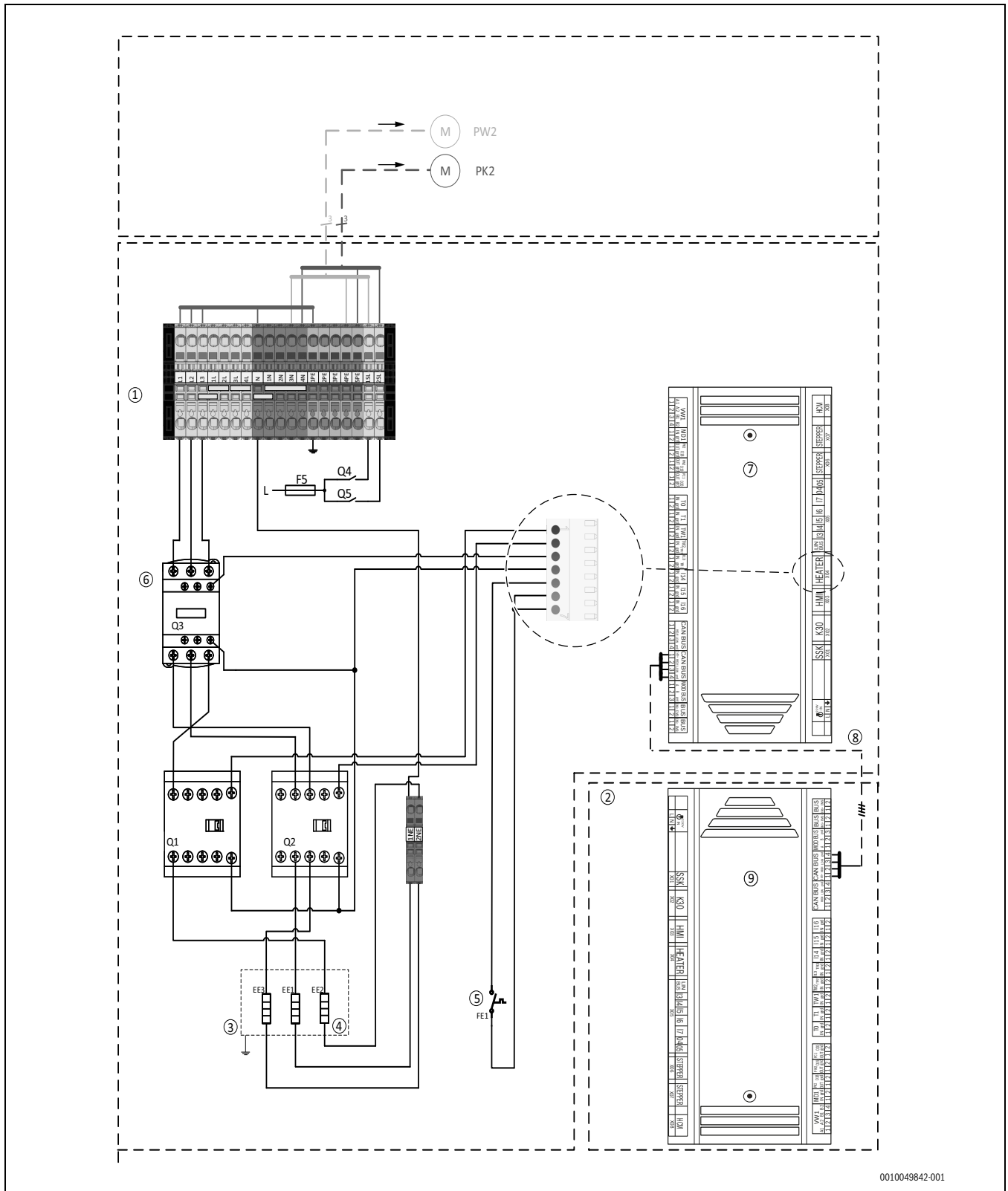
Bild 57 Spannungsversorgung Inneneinheit
