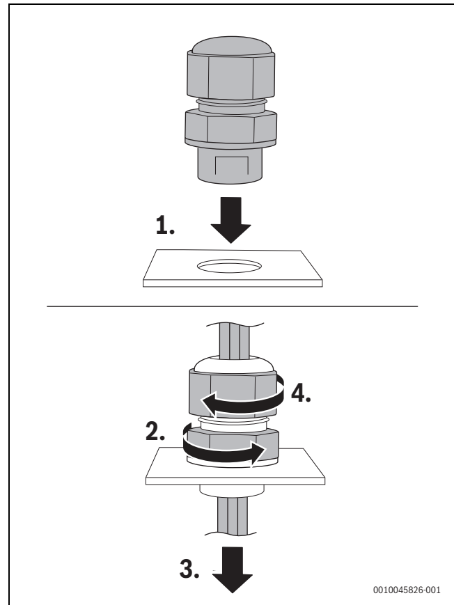
Bild 31 Kabelverschraubungen einsetzen
