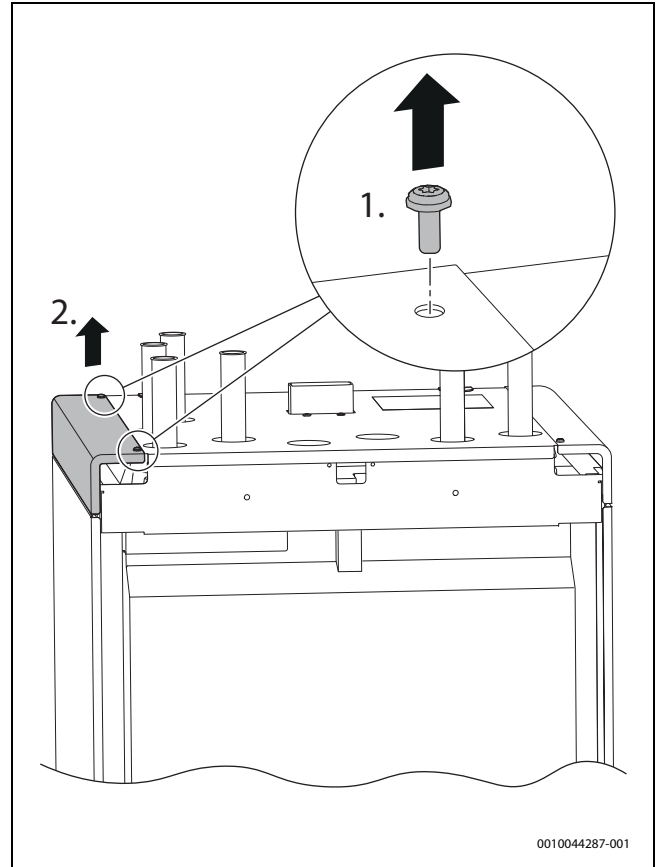
Bild 28 Rückansicht: Ecken mit Befestigungsschrauben
