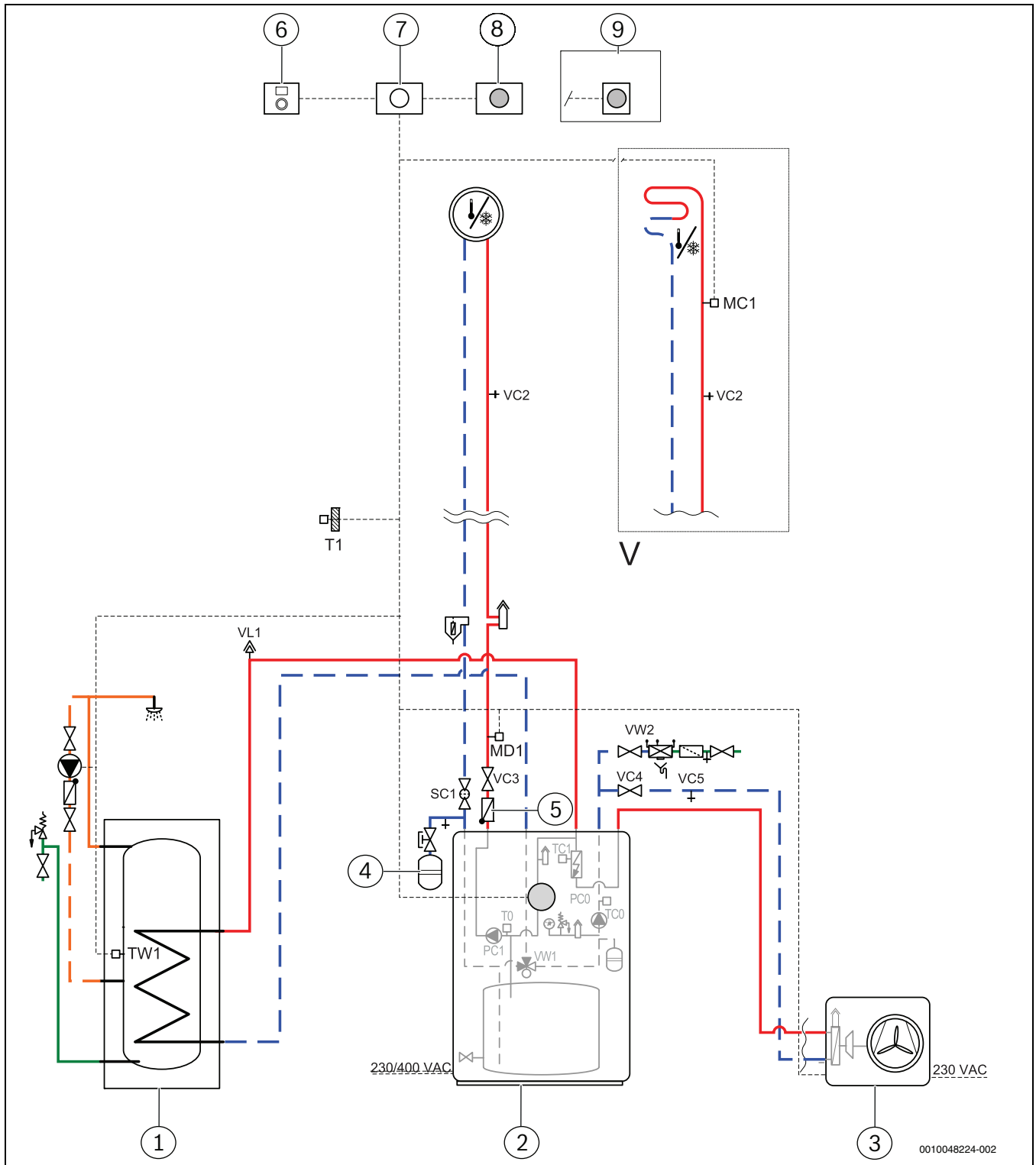
Bild 60 Anlage mit Außeneinheit, Inneneinheit mit integriertem Zuheizler, Pufferspeicher und einem ungemischten Heizkreis
