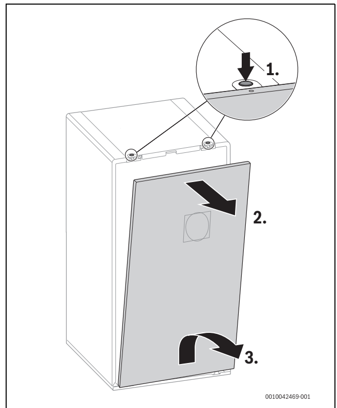
Bild 12 Vorderteil der Verkleidung abnehmen
