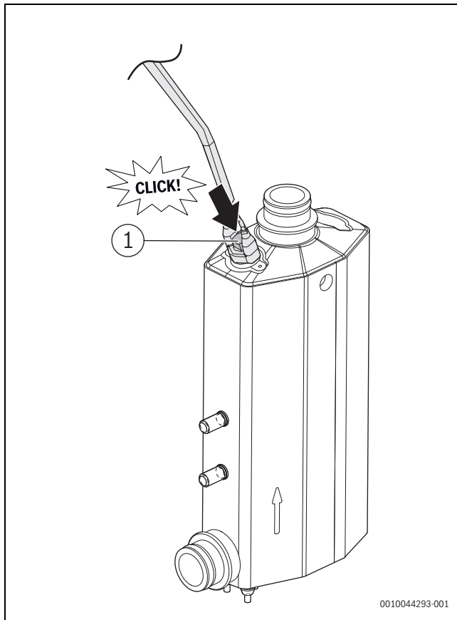
Bild 49 Elektrischer Zuheizer
