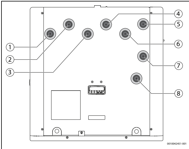
Bild 18 Hydraulische Anschlüsse
