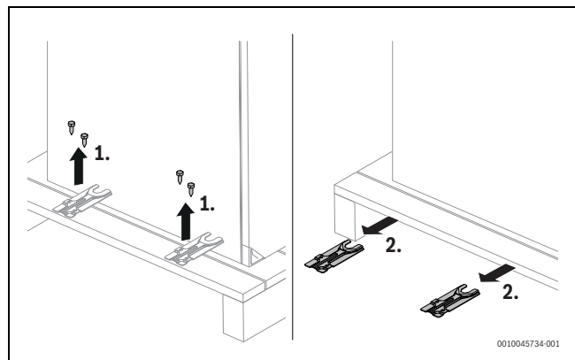
Bild 8 Transportsicherungen entfernen
