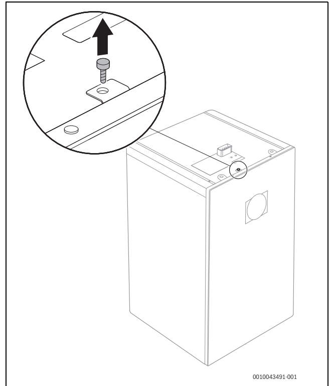
Bild 11 Sicherungsschraube lösen
