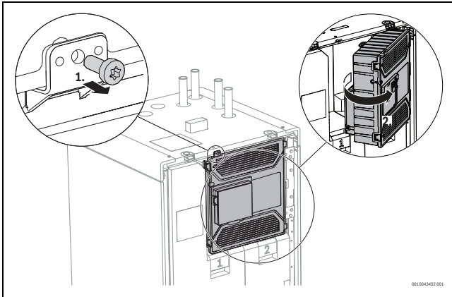
Bild 50 Elektronikbox
