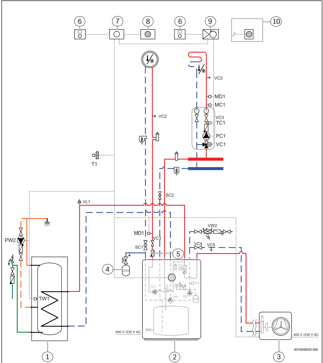
Bild 61 Anlage mit Außeneinheit, Inneneinheit mit integriertem Zuheizter und Pufferspeicher, einem ungemischten und einem gemischten Heizkreis
