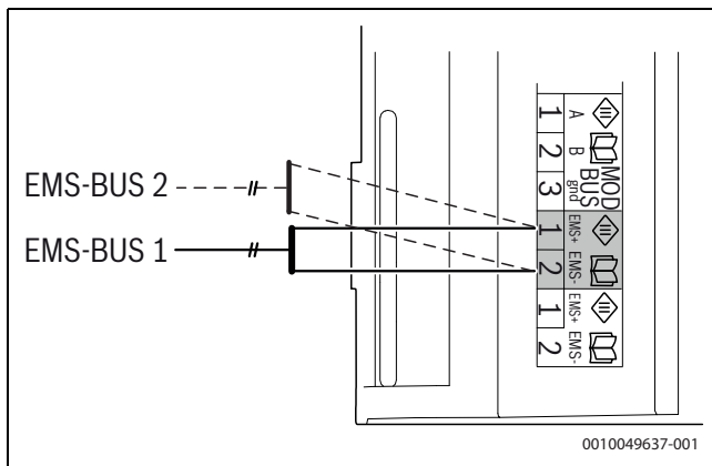
Bild 41 Anschluss mehrerer EMS-BUS-Kabel im Anschlussbereich XCU-THH für Steuer- und Fühlerkabel
