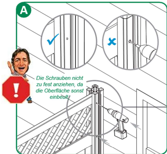
A -Schrauben Sie eine 3,5-Zoll-Schraube durch die Pfosten in die Riegel
