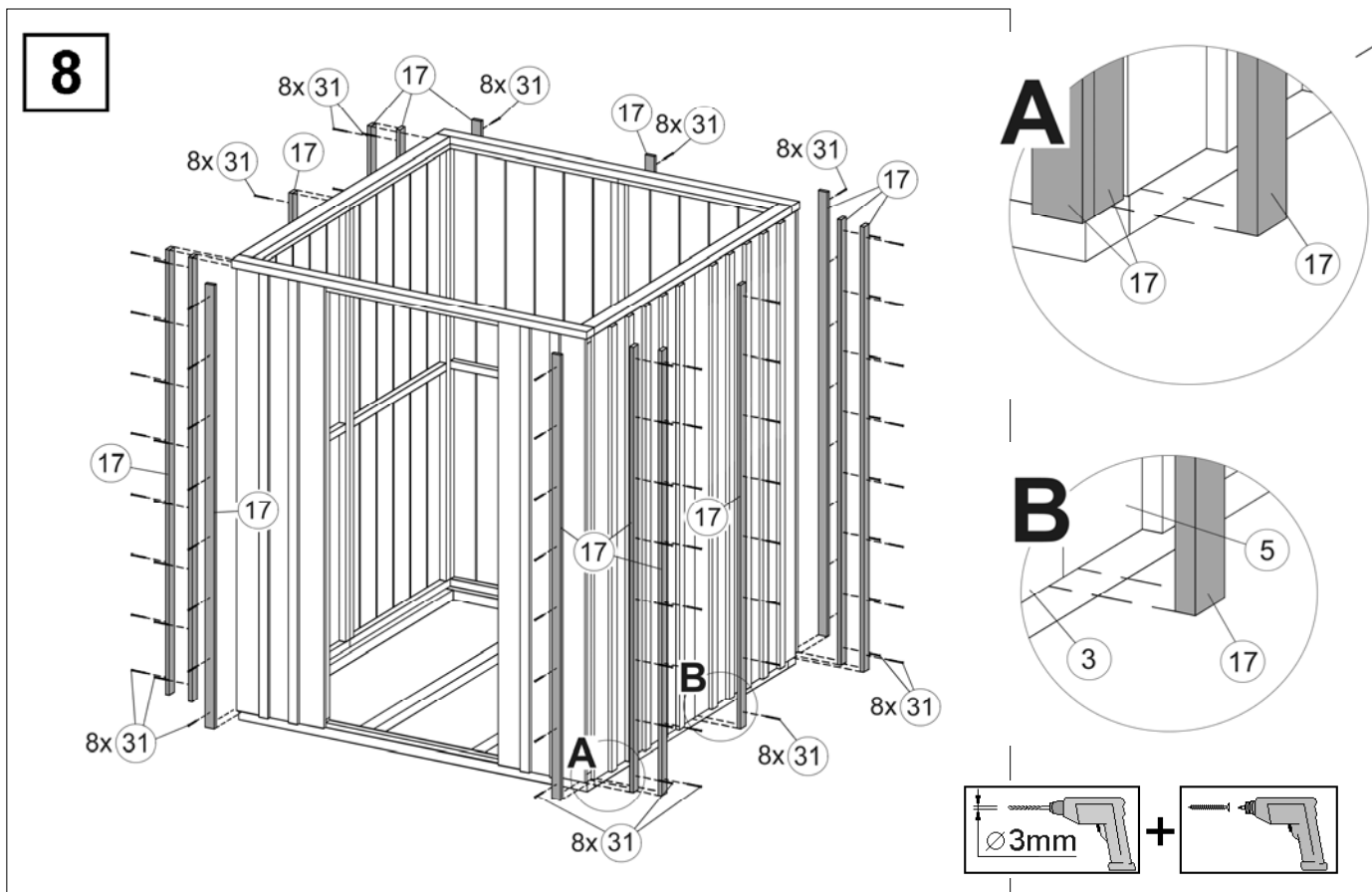
Abbildung Art.-Nr.: 348.1617
