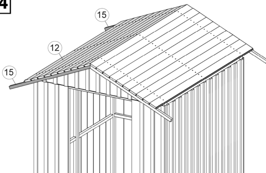
Abbildung Art.-Nr.: 348.1617
