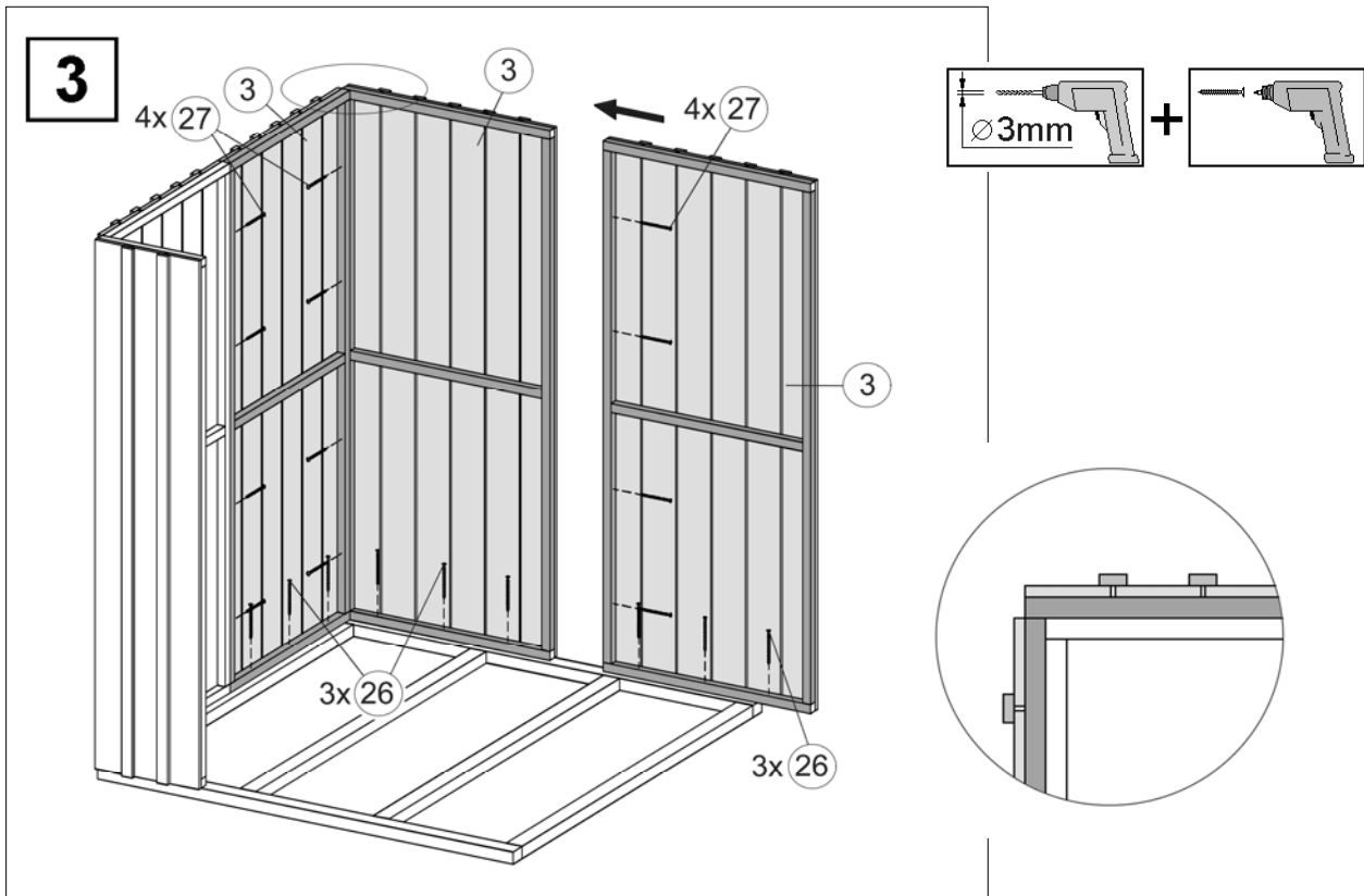
Abbildung Art.-Nr.: 348.1617
