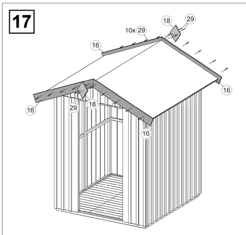
Abbildung Art.-Nr.: 348.1617
