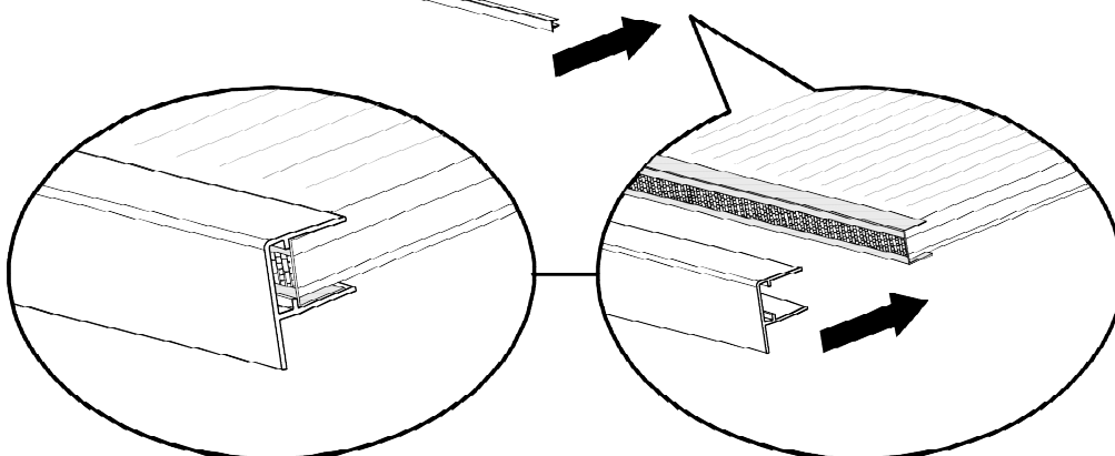
Pos 6 Kondensprofil
