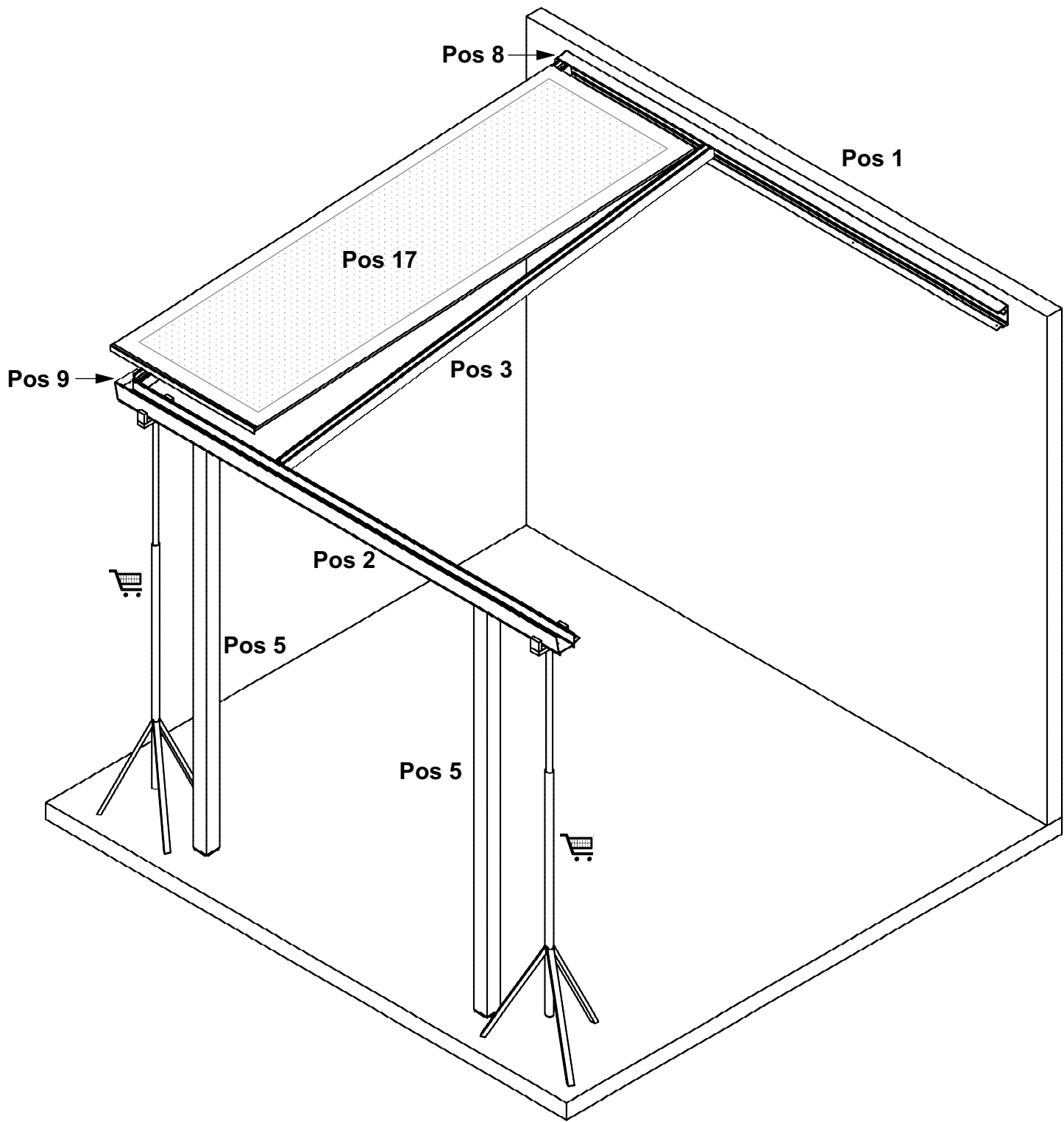
Detailskizze Montage Träger an Rinne
