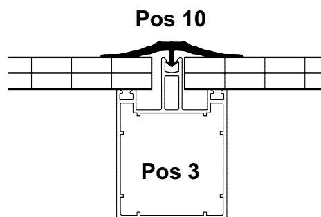
Detail Zwischenträger
