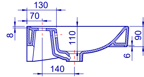
A-A KESİTİ
