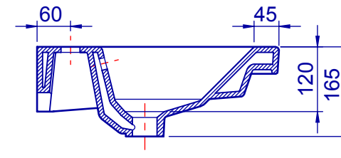
A-A' KESİTİ
