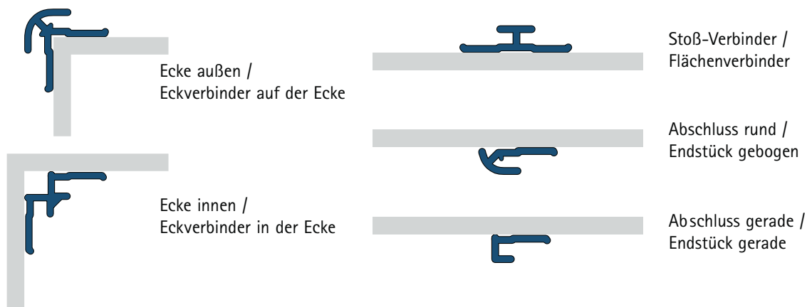
Beispiel 1: Einbau auf gerade Wand, mit gerundetem und geradem Abschlussprofil
