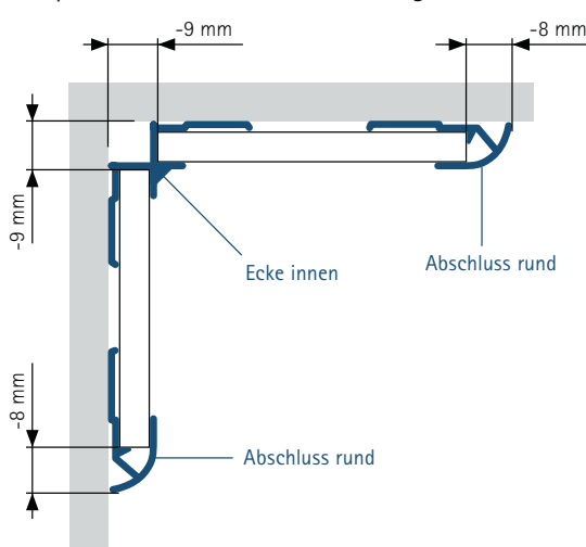
Beispiel 3: Einbau in einer Ecke, mit gerundeten Abschlussprofilen.
