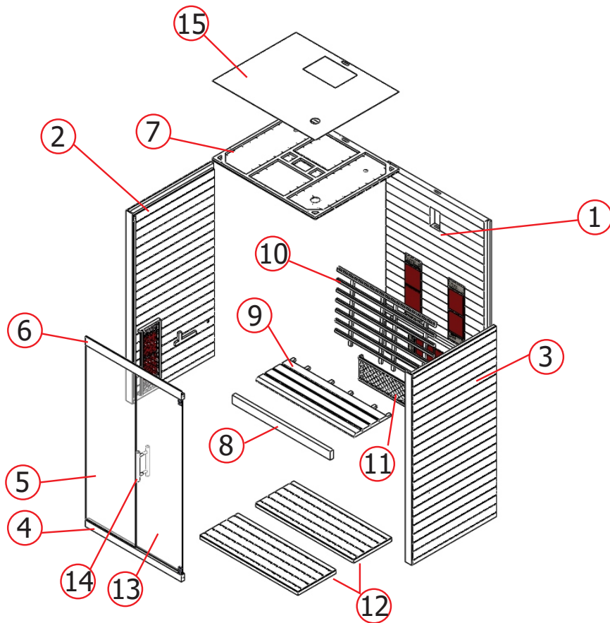
Kabinen-Einzelteile (Variationen möglich)
