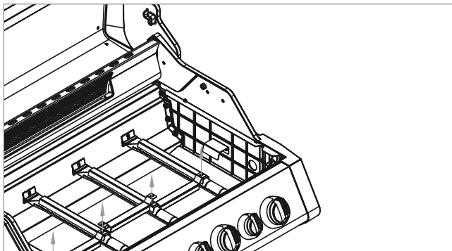
1. Schrauben lösen und Befestigung abheben.
