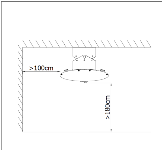
Plafond montage:
