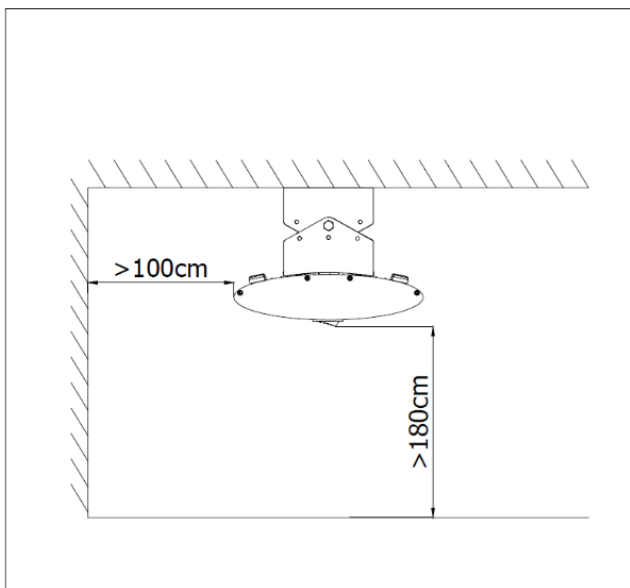
Deckenmontage:
