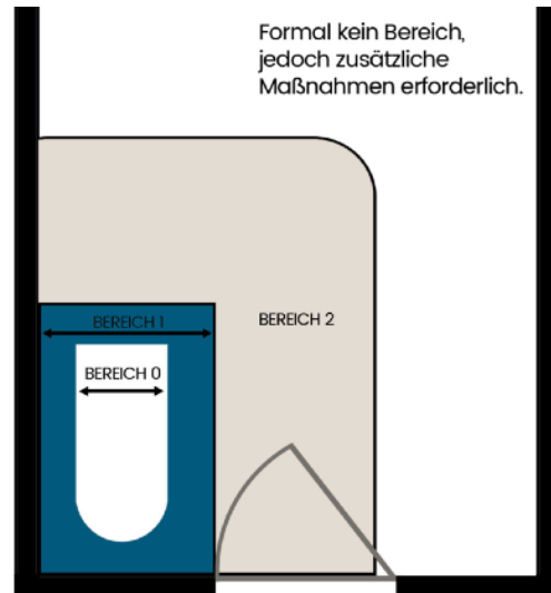
Abb. 02: Montage in Feuchträumen und Bädern
