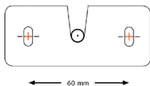
Abb. 03: Bohrlöcher
