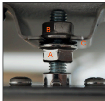
Abb. 07: Wandmontage
