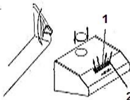
Recirculation mode
