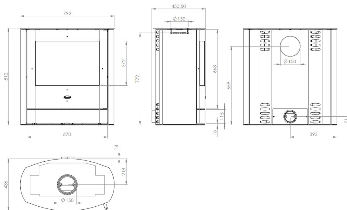
Abbildung 6 - Hauptmaße
