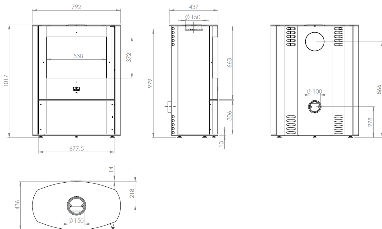
Abbildung 2 - Hauptmaße
