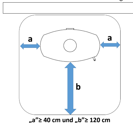
Abbildung 13 – Bodenplatte
