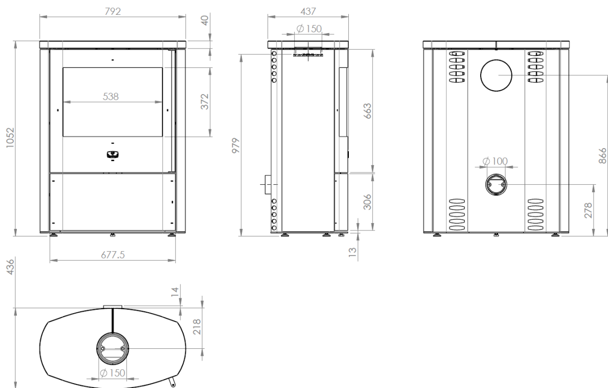
Abbildung 4 - Hauptmaße
