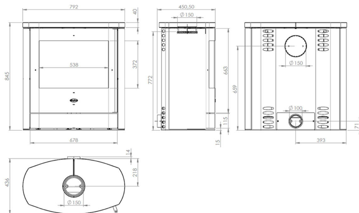
Abbildung 7 - Hauptmaße
