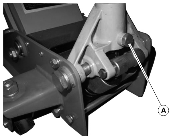
Abb. 5: Feststellschraube
