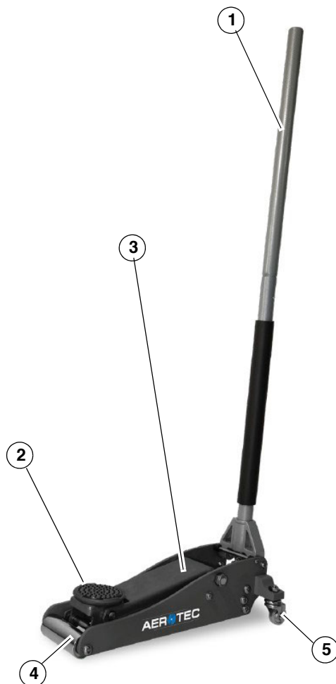
Abb. 3: Gerätebeschreibung ARHWA 1502
