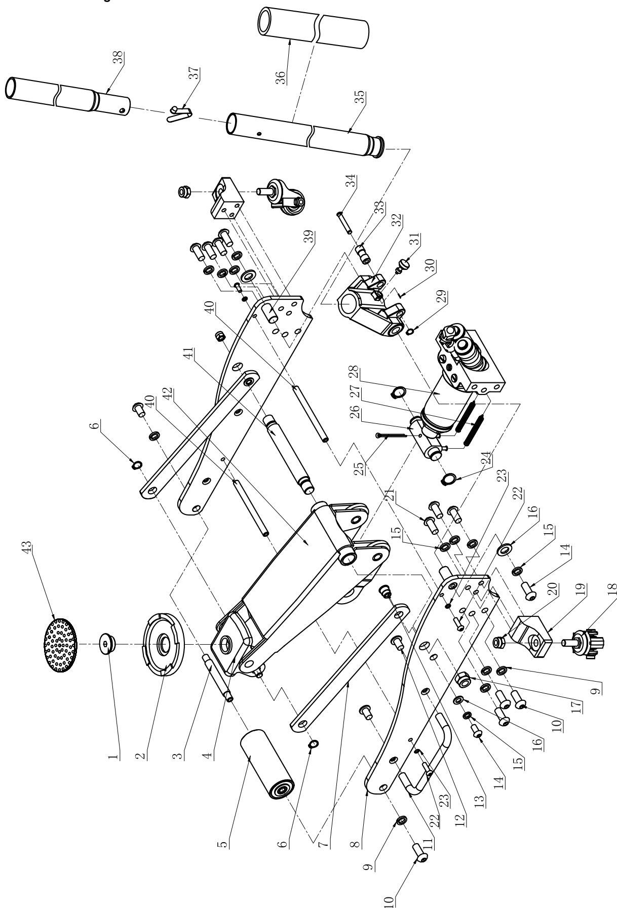
Abb. 9: Ersatzteilzeichnung ARHWA 1502
