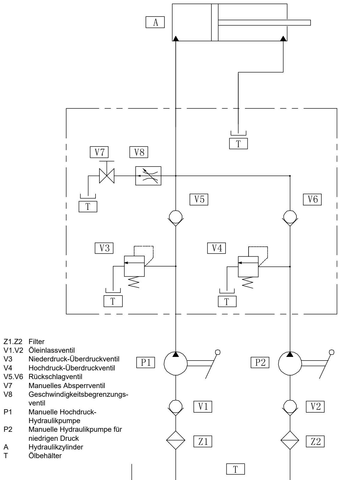
Abb. 10: Hydraulikplan
