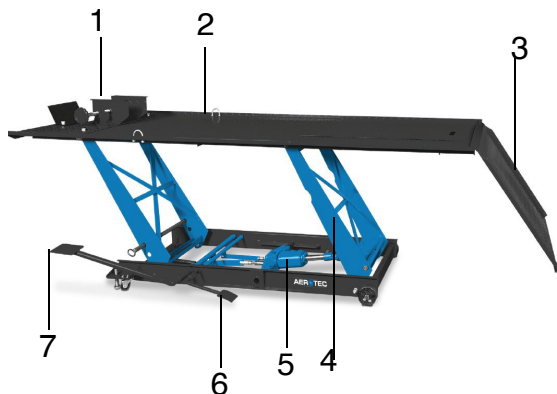
Abb. 3: Gerätebeschreibung MHB 455
