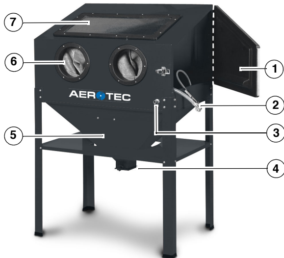
Abb. 3: Sandstrahlkabine ASK 2
