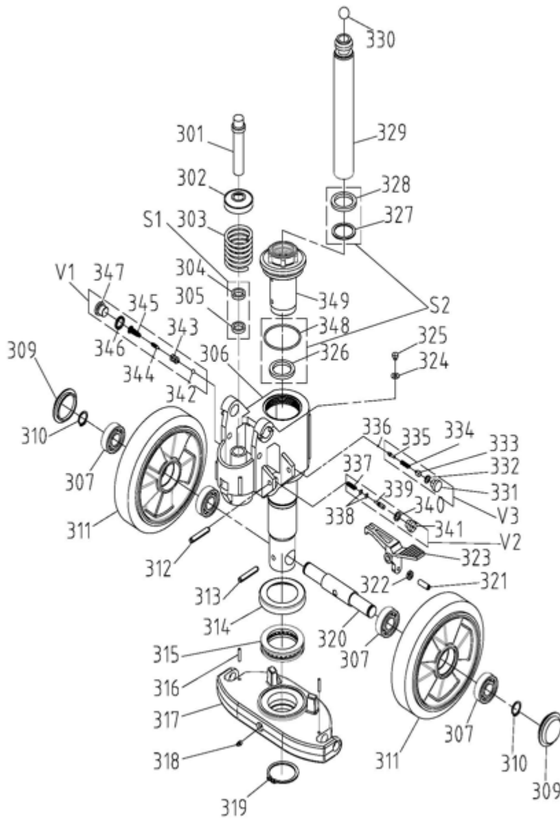
Abb. 9-3: Ersatzteilzeichnung 3
