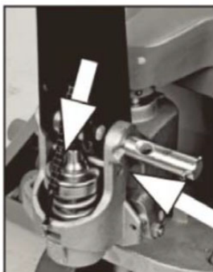
Abb. 5-2: Deichsel auf das Pumpengehäuse setzen
