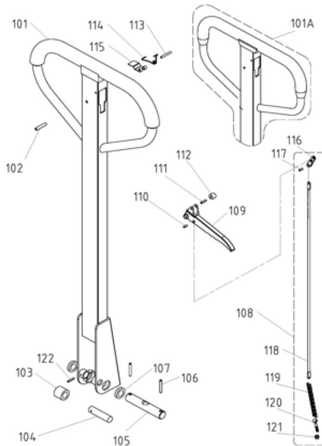
Abb.9-1: Ersatzteilzeichnung 1
