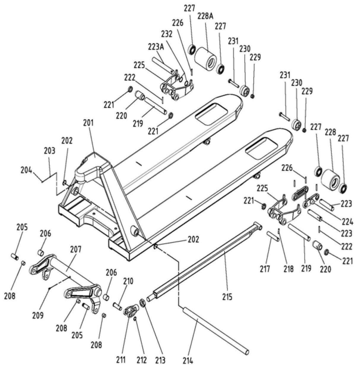
Abb.9-2: Ersatzteilzeichnung 2
