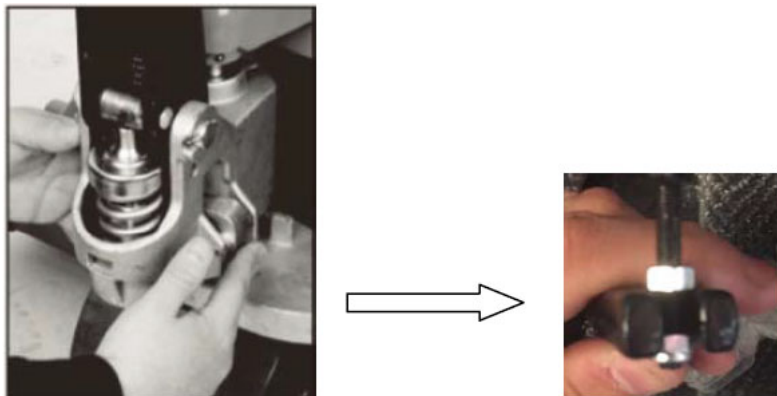
Abb. 5-6: Positionieren der Einstellmutter oberhalb des Hakens
