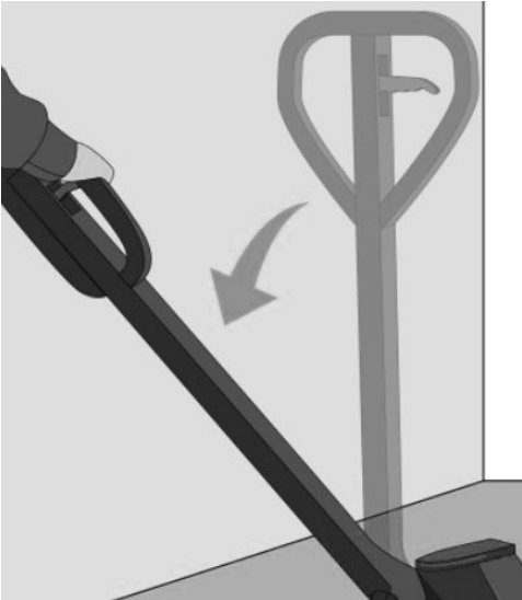
Abb.7-1: Hydrauliksystem entlüften
