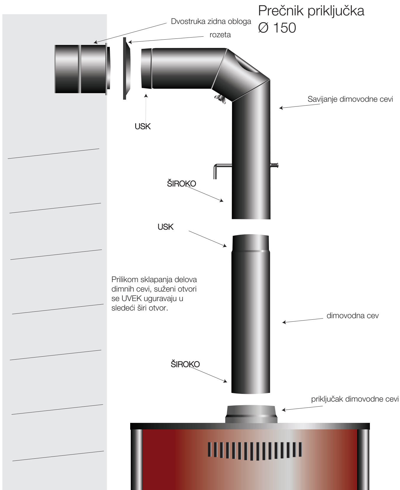
Slika 3 Povezivanje peći na drva sa dimnjakom
