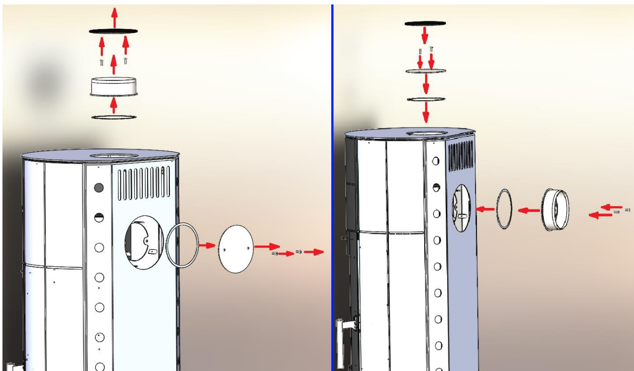
Figur 2 Ofbau vum Kamäinanschluss/Kamäindeckel
