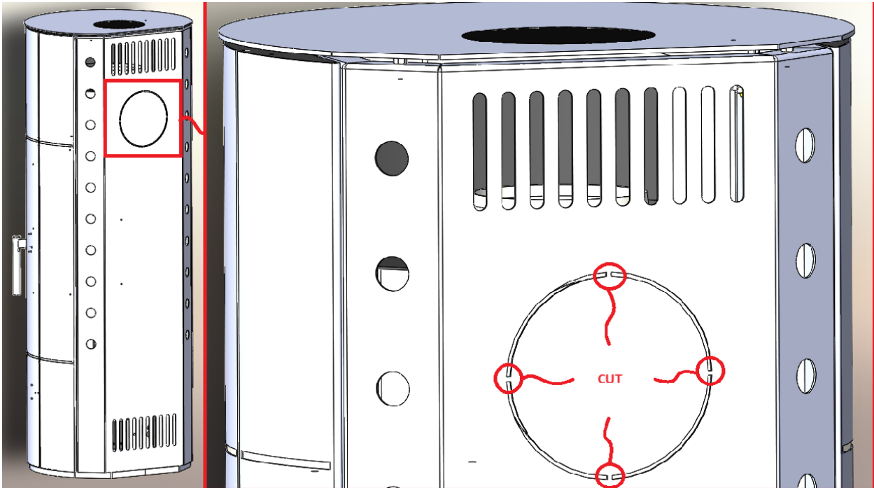
Figur 1 Schneiden vu mikrogeschweesste Verbindungen op der Récksäit vum Kamäin
