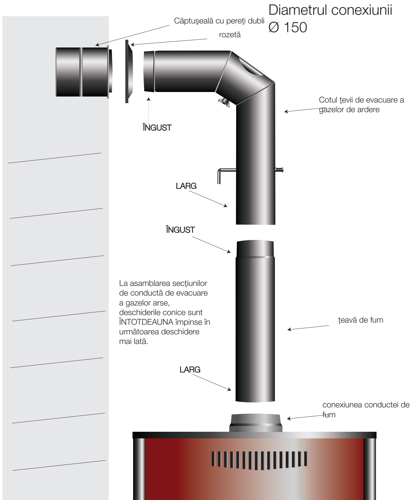
Figura 3 Conectarea sobei pe lemne la coș
