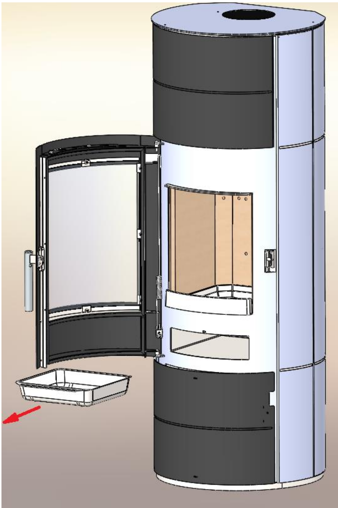
Figura 5 Svuotamento del cassetto della cenere
