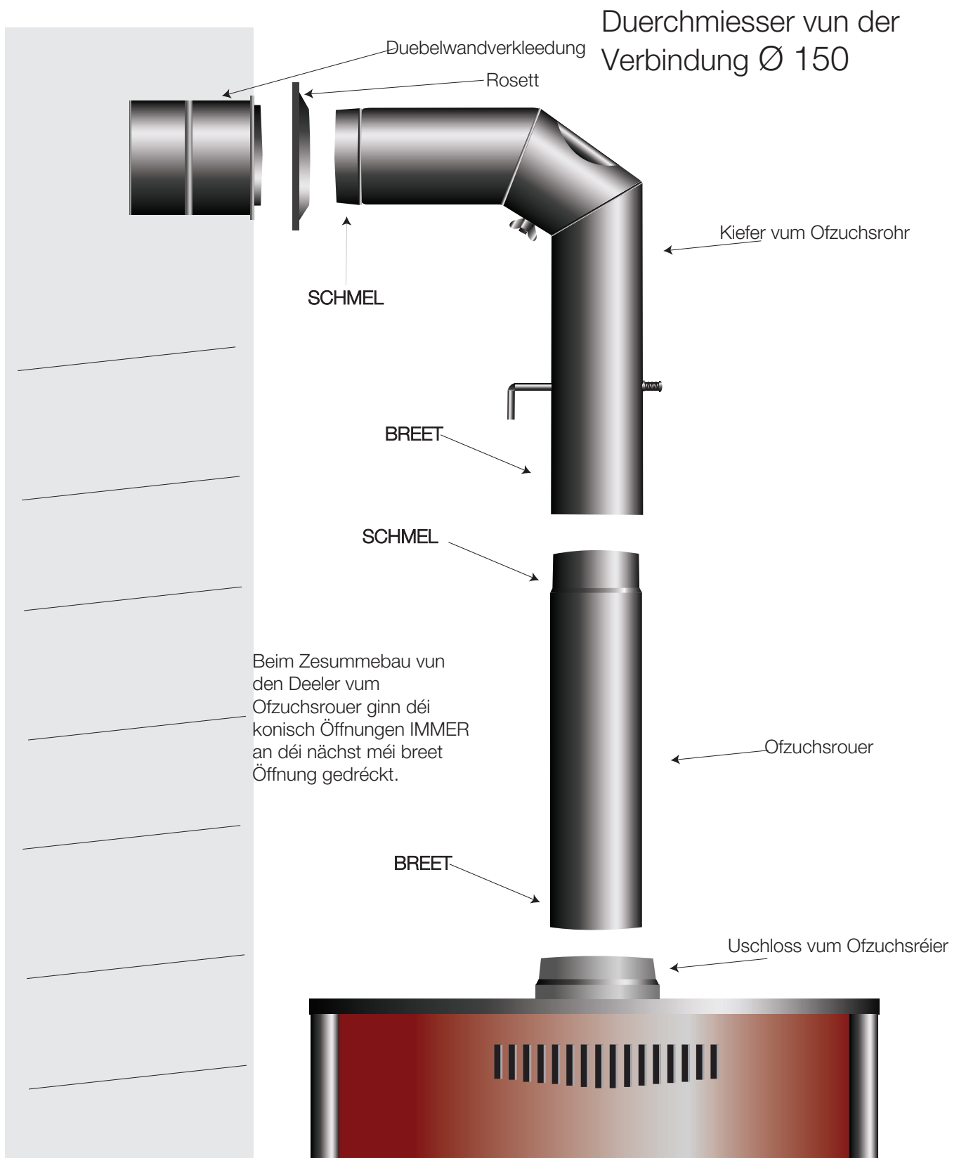
Figur 3 Uschloss vum Uewen un de Kamäin
