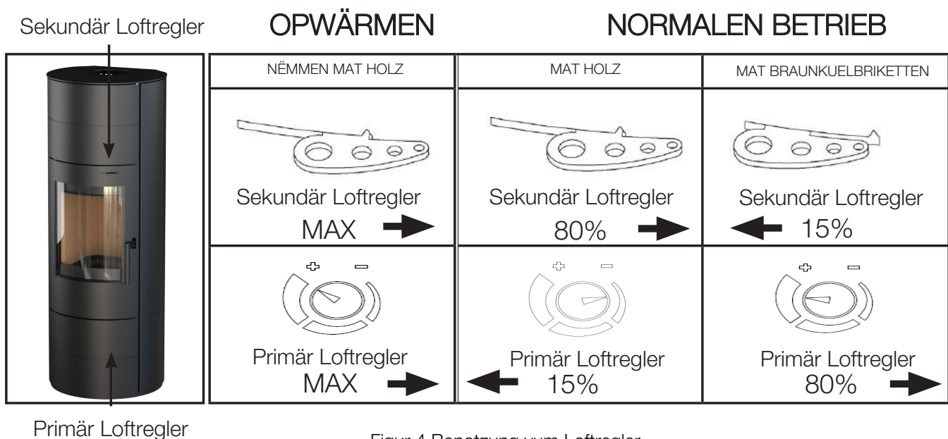
Figur 4 Benetzung vum Loftregler
