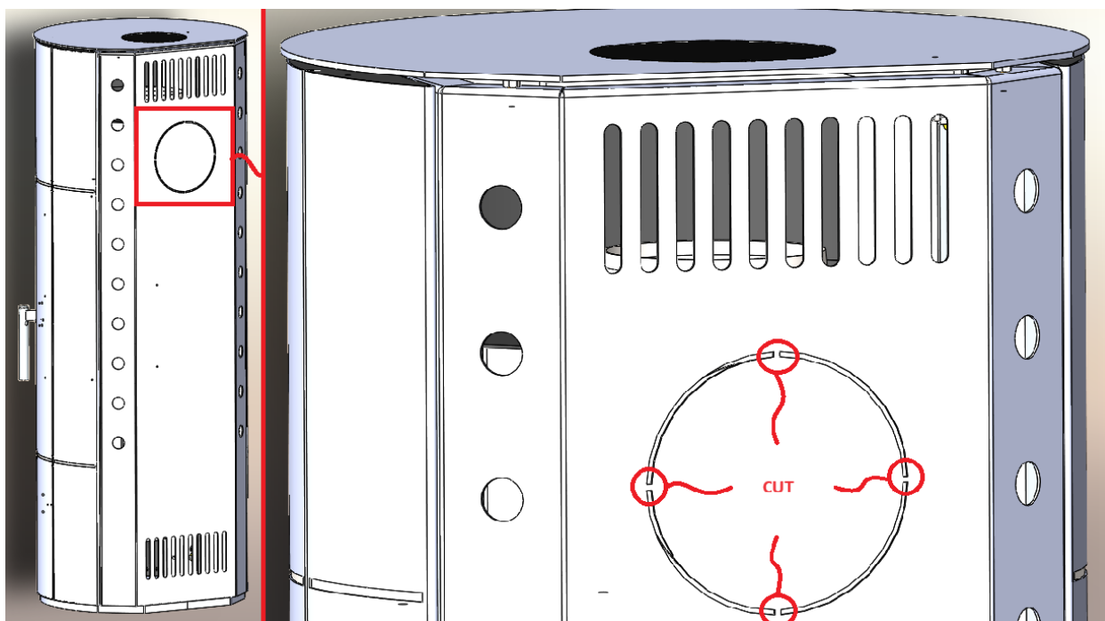
Figura 1 Sezionamento delle microconnessioni sul retro
