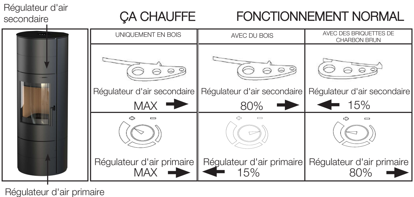
Figure 4 Utilisation du régulateur d'air
