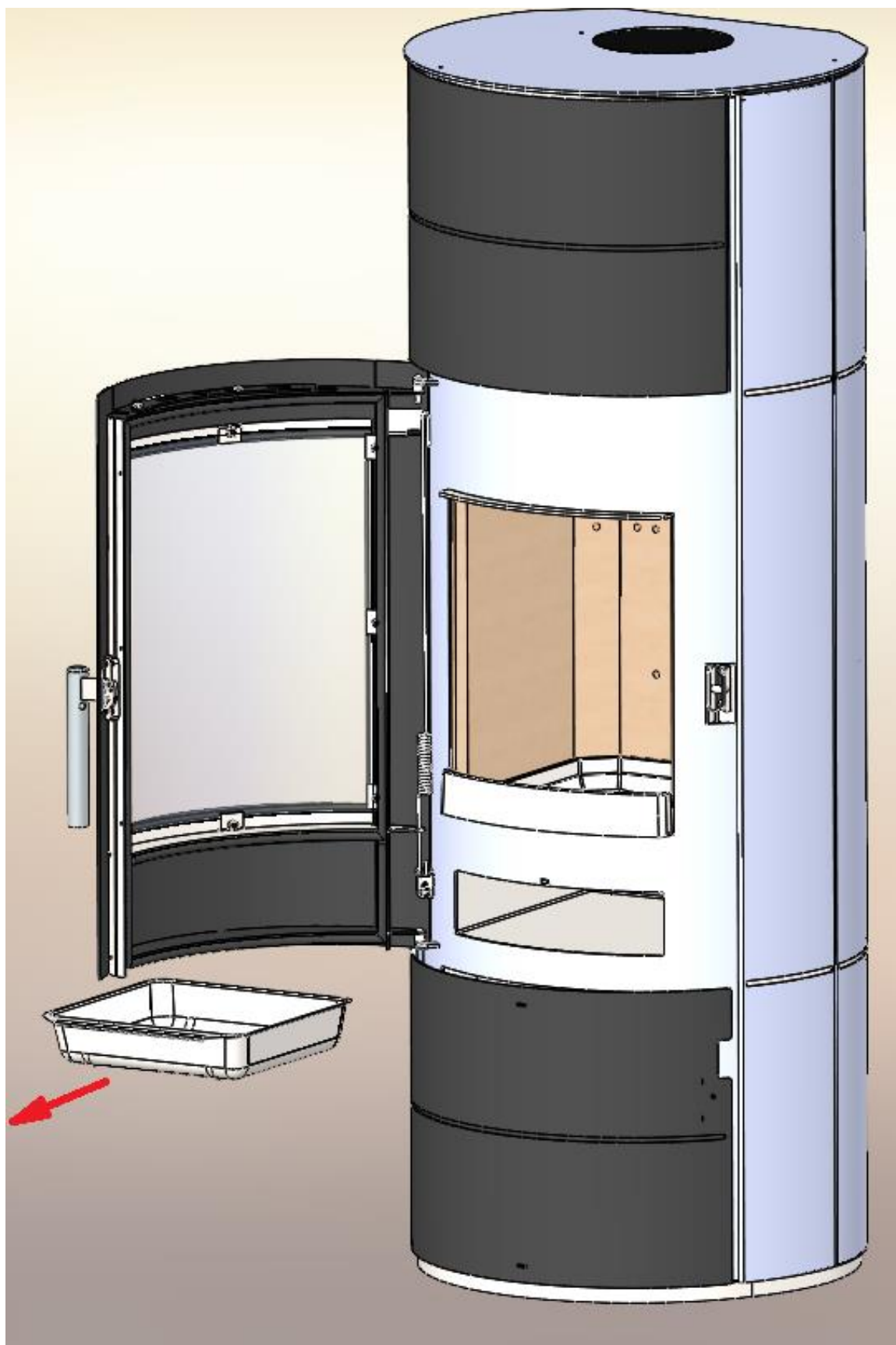
Slika 5 Pražnjenje posude za pepeo
