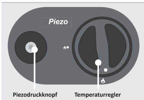
Abb. 5a: Bedienfeld (Modelle ohne Thermostat)
