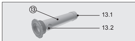
⑬ Tubo de llenado con parallamas KITO® para el llenado (13.1) y la desaireación (13.2)
