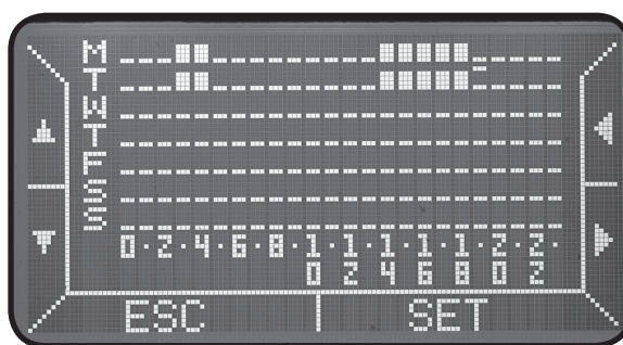
Abb. 10b: Display-Anzeige SET TIMER, programmiert
