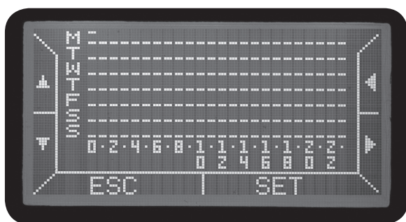
Abb. 10a: Display-Anzeige SET TIMER
