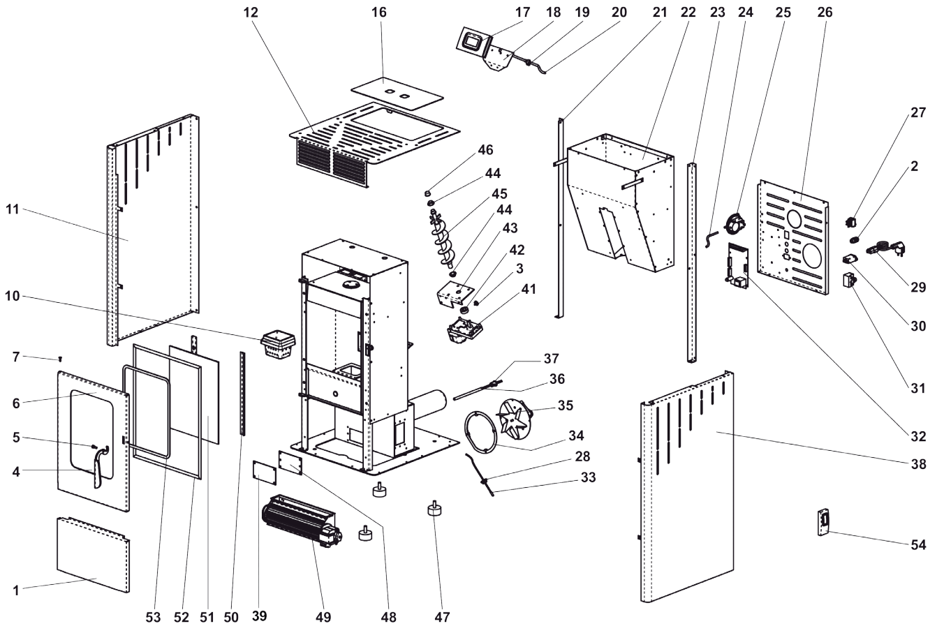
Abb. 16 : Explosionszeichnung
